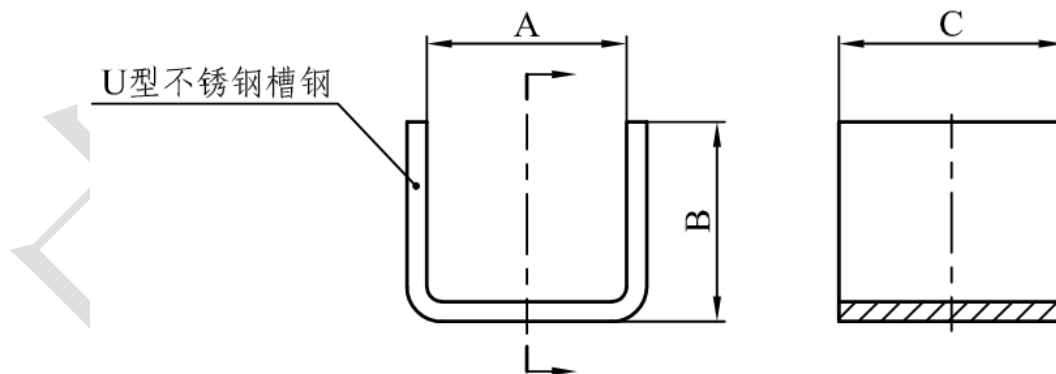
图 5 U 型槽钢加工示意图
