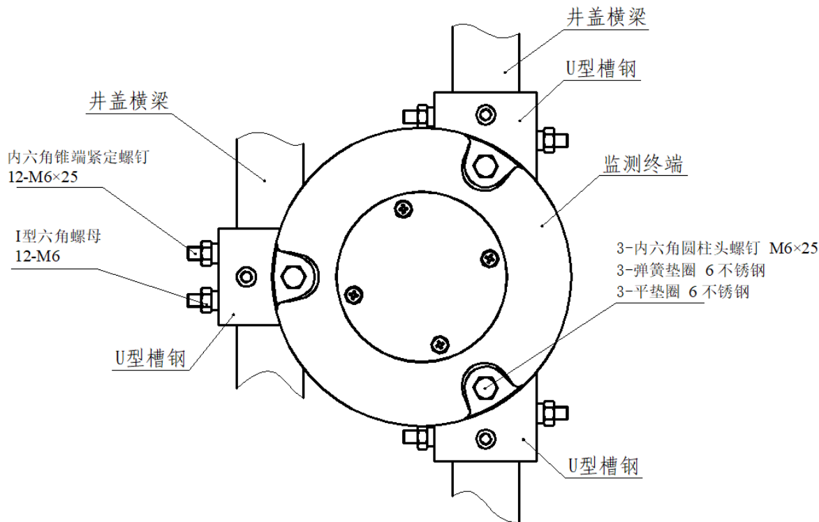
图 8 非金属复合材料井盖监测终端安装示意图（安装附件 CS-iTWM-A02）
