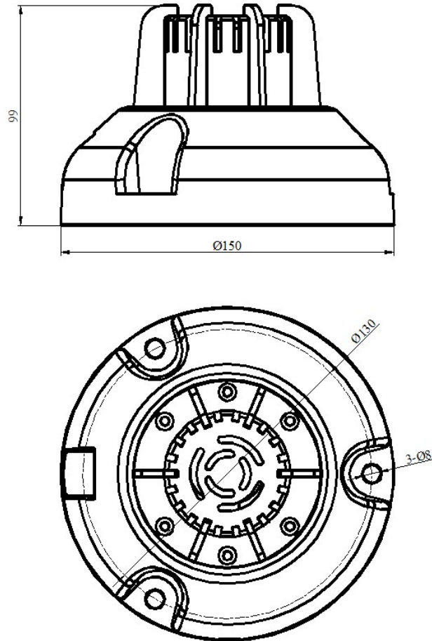
图 2 终端尺寸图
