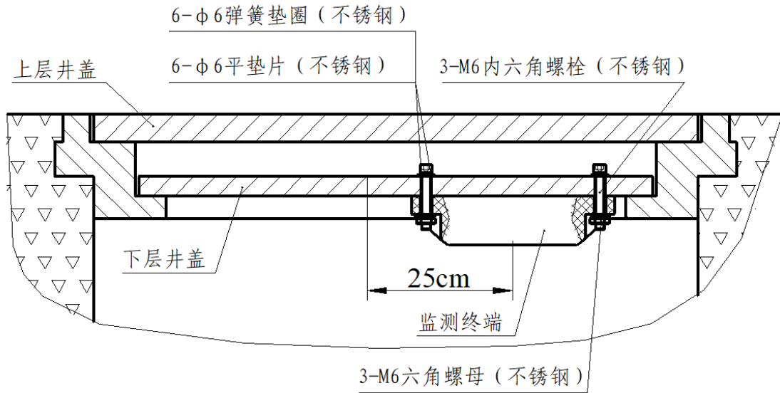
图 3 双层井盖安装示意图（安装附件 CS-iTWM-A03）
