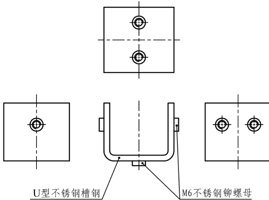
图 6 铆螺母安装示意图
