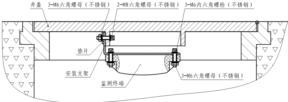
图 11 雨水球墨铸铁材料井盖安装示意图（安装附件 CS-iTWM-A01）
